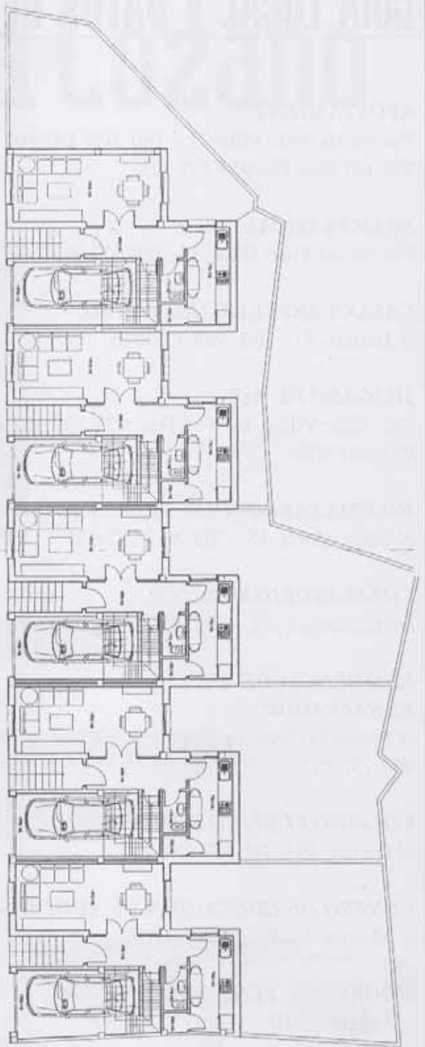
Planta General
